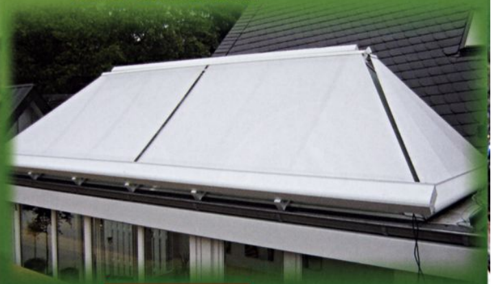
Zwei Vieleckmarkisen mit gemeinsamer Variette II-Kassette und Ausfallprofil sowie eine Dreiecksbeschattung
